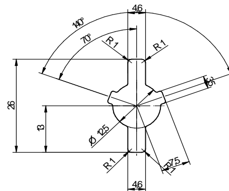
Skizze 2: Schlüsselträgerführung 86102
