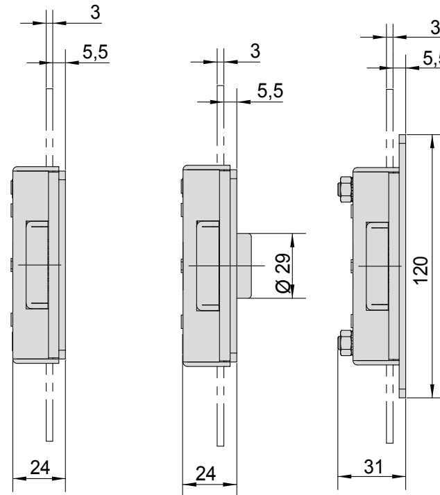
Schloss mit Montagedecken / Lock with mounting covers
