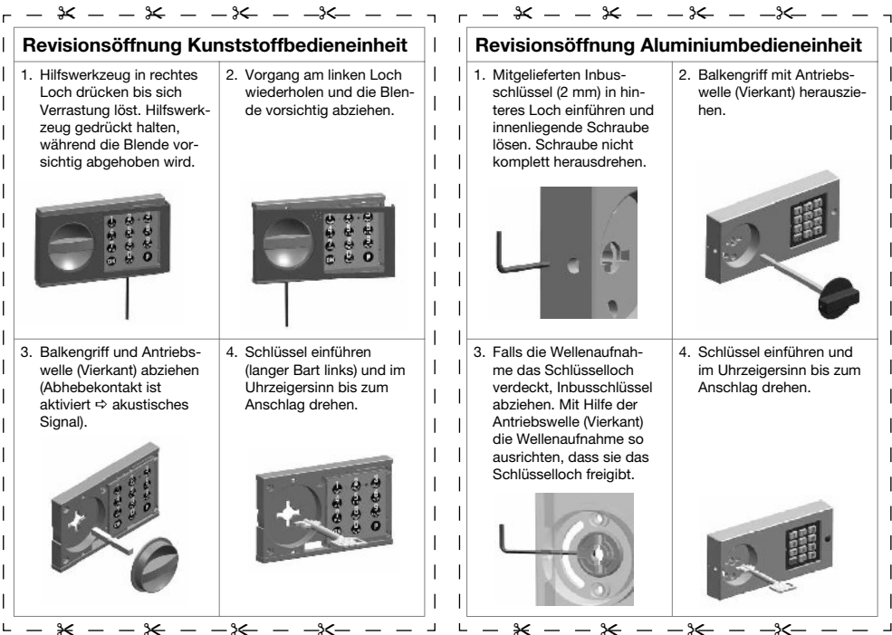
Abb. 6: Kunststoffbedieneinheit
